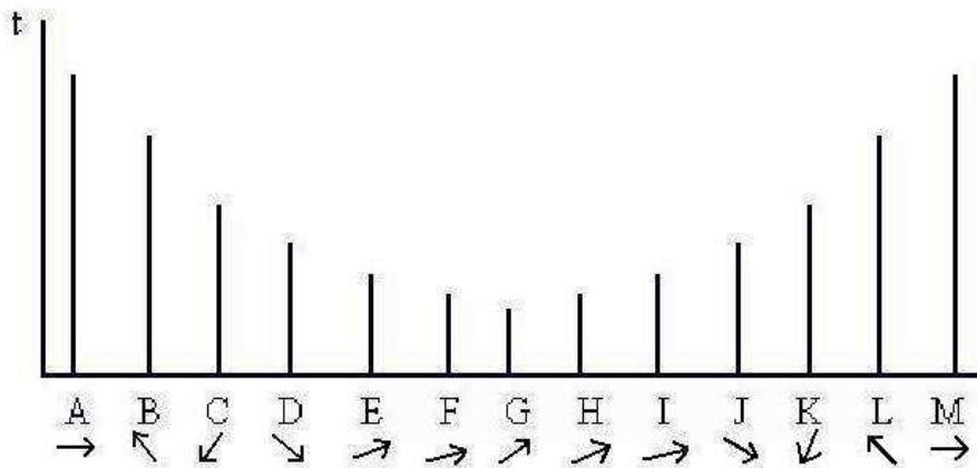
Figura 2.3: A cada caminho possível é associado uma seta de um certo tamanho fixado. A direção da seta varia a medida que o tempo muda. Nesse sentido, somar amplitudes está associado a somar setas. Assim vemos que a maior contribuição para a soma total ocorre entre E e I, onde as direções são quase as mesmas porque os tempos dos caminhos naquela região são quase os mesmos.
