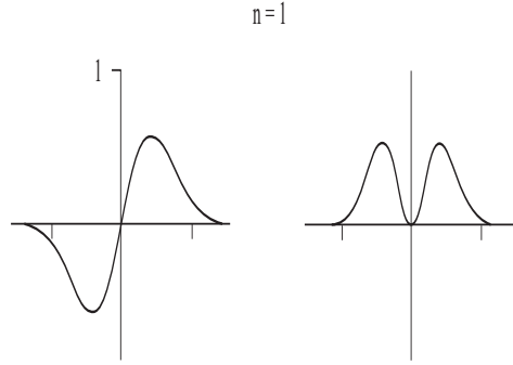
Figura 1.10: Seja \psi_1 a segunda autofunção do oscilador harmônico. A esquerda seu gráfico e a direita o gráfico de |\psi_1|^2
