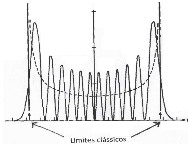
Figura 1.8: A linha pontilhada descreve o tempo de ocupação assintótica da partícula no nível de energia E segundo a Mecânica Clássica. A linha cheia descreve a densidade |\psi|^2 associada a um estado \psi que se encontra neste mesmo nível de energia E = E_{20} = (20 + 1/2)w\hbar . Note que existe uma probabilidade positiva de se encontrar a partícula fora da região clássica. Isto descreve o fenômeno do tunelamento. Ver também figuras 1, 2 e 3 em [144].
