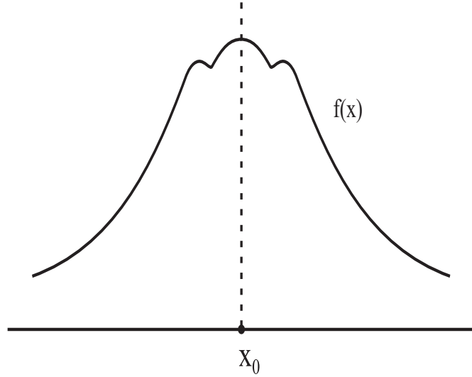
Figura 1.13: Densidade f(x) com dados que possuem forte concentração em torno da média.
