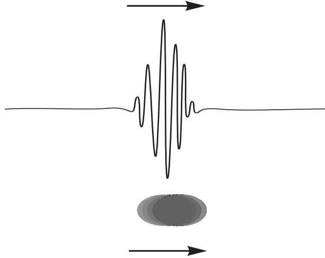
Figura 1.5: A transformada de Fourier \hat{\psi}(p) de um estado \psi tal que aproximadamente vale |\psi(x)|^2 = \cos(\alpha x) . A região mais escura descreve a área de maior probabilidade de encontrar o momento p do estado \psi (Wikipedia)
